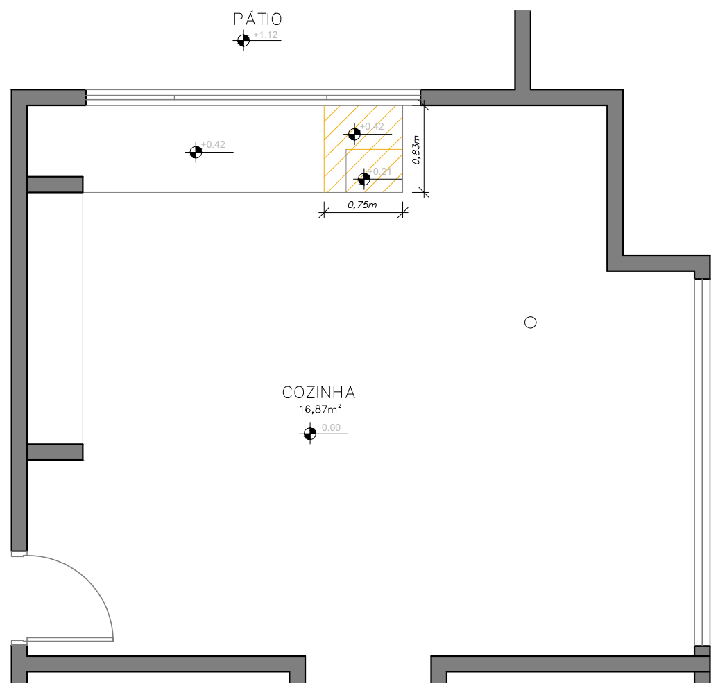
PLANTA BAIXA - SITUAÇÃO ATUAL ESC.: 1:50
