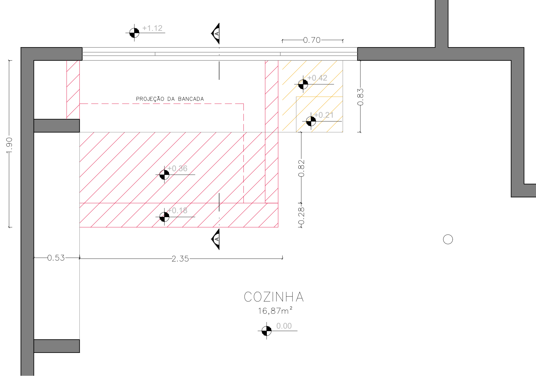
PLANTA BAIXA - REFORMA ESC.: 1:25
