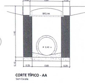
CORTE TÍPICO - AA Sem Escala
