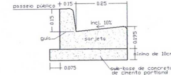
CORTE TÍPICO - GUIA E SARJETA Sem Escala
