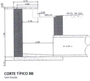
CORTE TÍPICO BB Sem Escala
